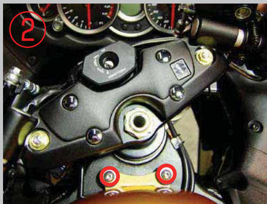
キャップボルト M6×35mm 2本
